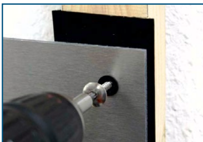
Abb. 12 - Schraubvorgang
